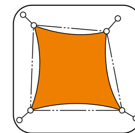
Viereck
