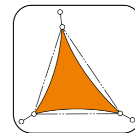
Dreieck
