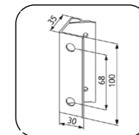
Montagewinkel auf Blendrahmen
