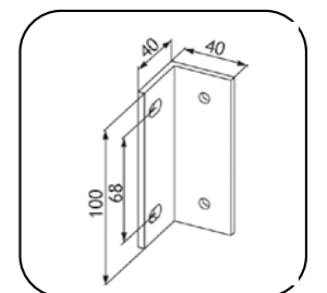
Laibungswinkel
